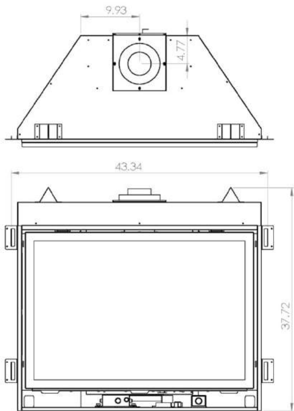
TOP VENT
